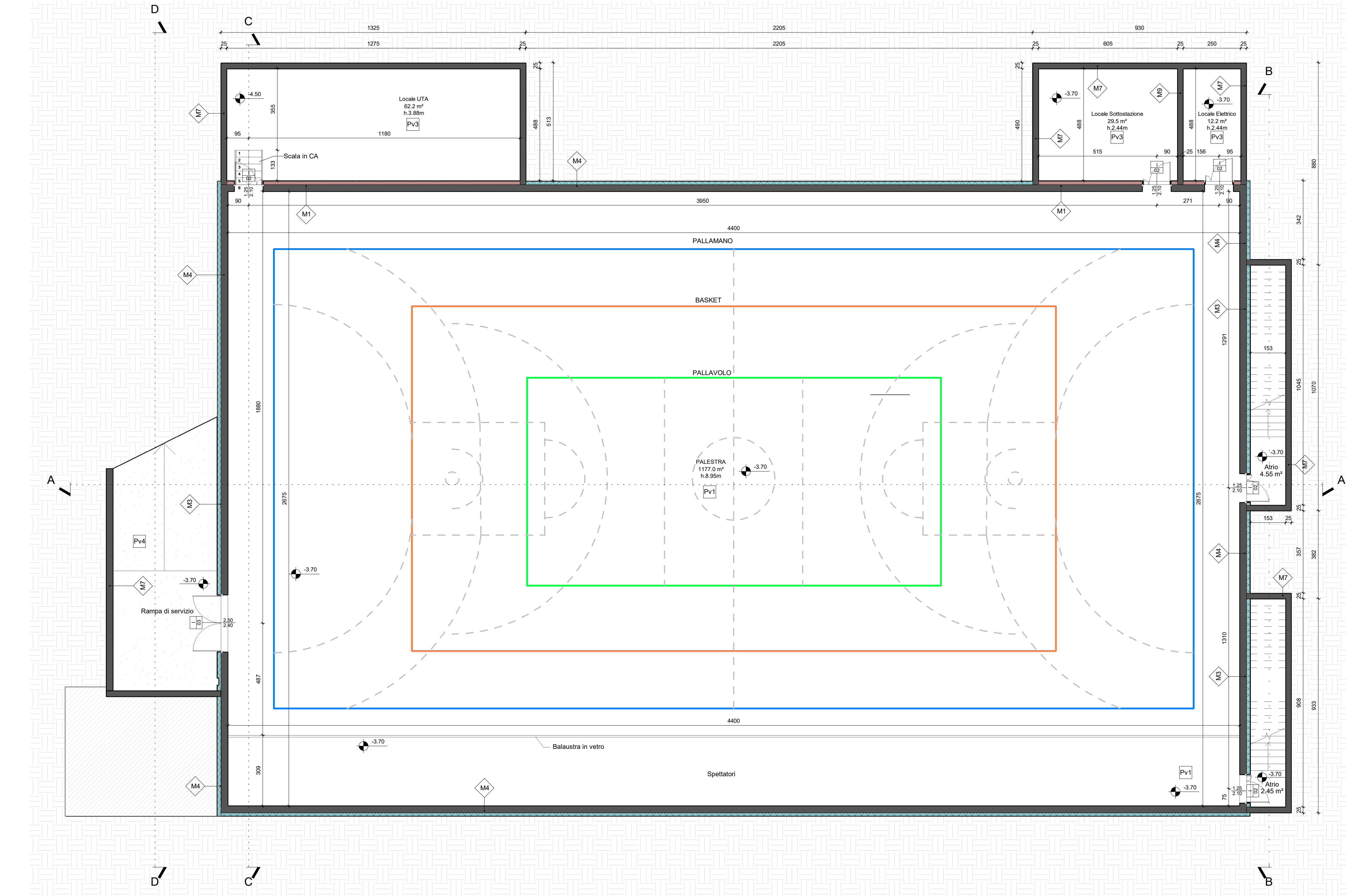
PIANTA PIANO INTERRATO
